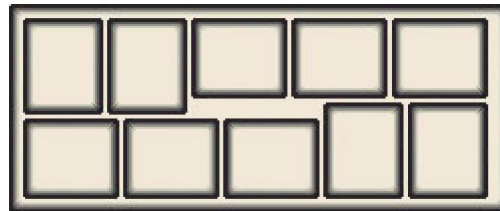
Рисунок 1б. Расположение финских паллет в контейнере 20DV (10 штук).
