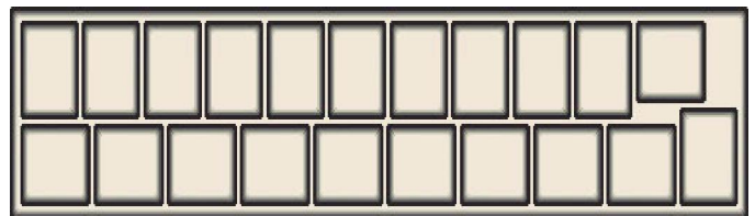
Рисунок 2б. Расположение финских паллет в контейнере 40DV/40HC (21 штука).
