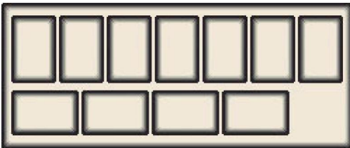
Рисунок 1а. Расположение европаллет в контейнере 20DV (11 штук).
